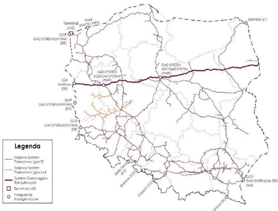
Mapa 43 Krajowy System Przesyłowy, którego operatorem jest GAZ-SYSTEM wraz z lokalizacją połączeń transgranicznych (stan na dzień 31.12.2024 r.)
