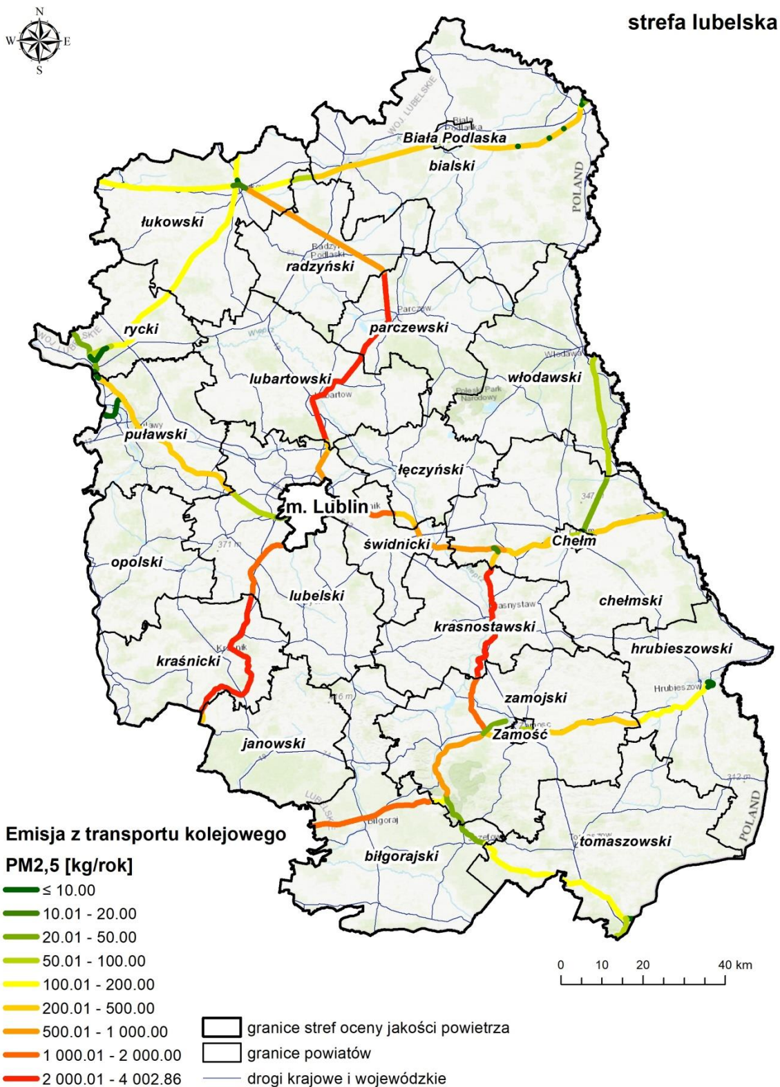
Rysunek 39. Emisja pyłu zawieszonego PM 2,5 z innych źródeł (kolej) 94
