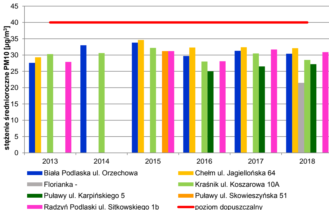
Rysunek 5. Stężenie średnioroczne pyłu zawieszonego PM10 notowane na stacjach pomiarowych w strefie lubelskiej w latach 2013-2018 41
