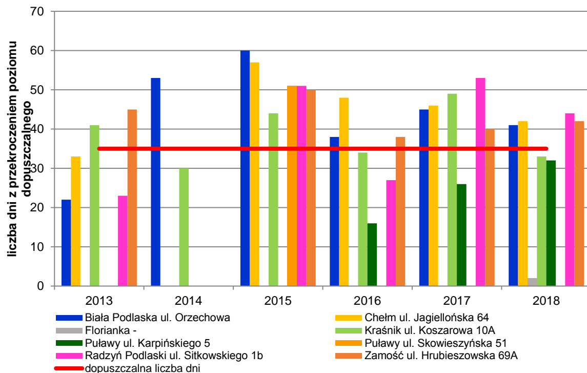
Rysunek 4. Liczba dni z przekroczeniem dopuszczalnego stężenia 24 godz. PM10 w strefie lubelskiej w latach 2013-2018 40
