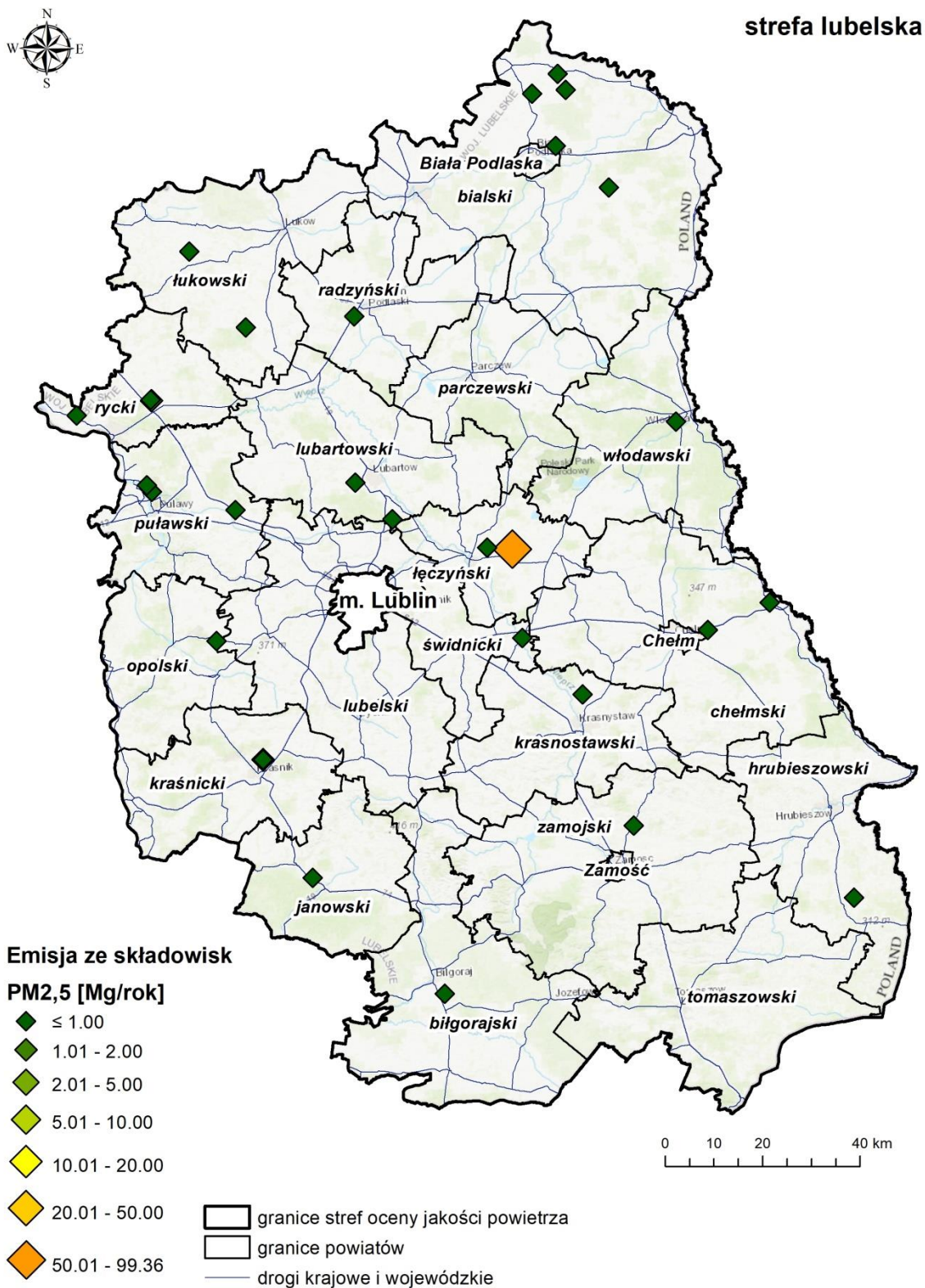
Rysunek 41. Emisja pyłu zawieszonego PM 2,5 ze składowisk odpadów 96
