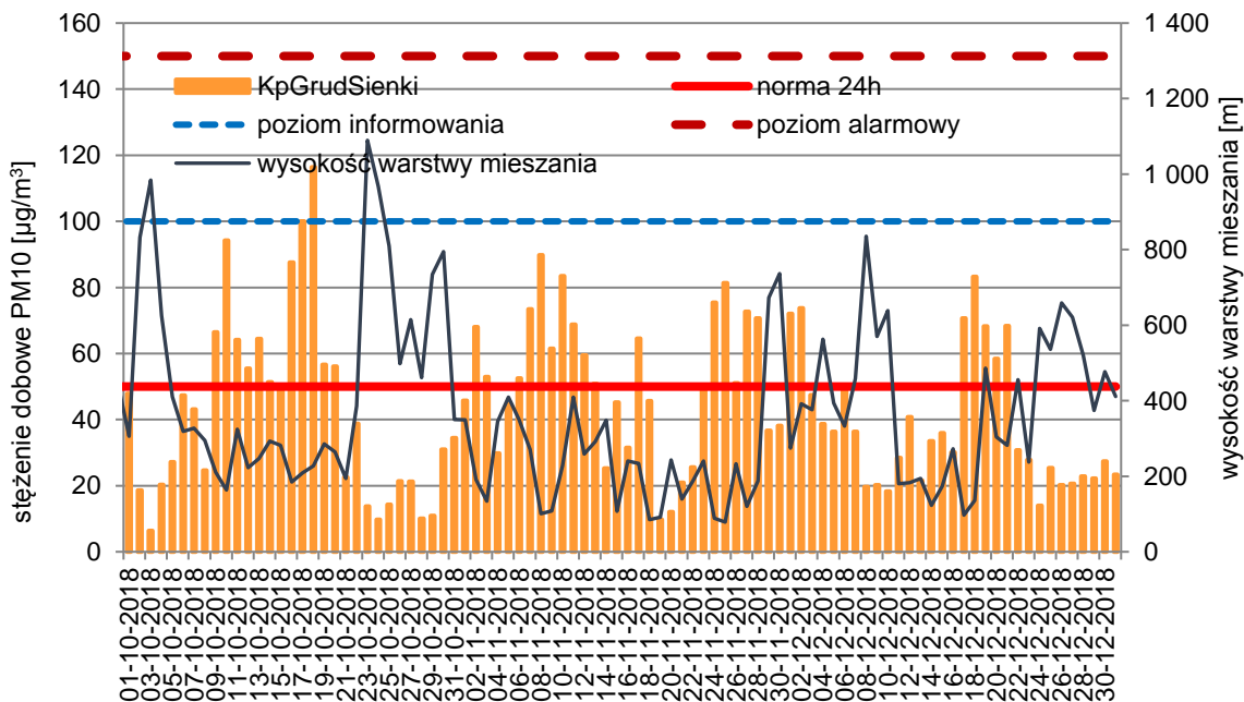
Rysunek 22. Porównanie przebiegu zmienności stężeń 24-godz. PM10 w IV kwartale 2018 r. w Puławach z wysokością warstwy mieszania
