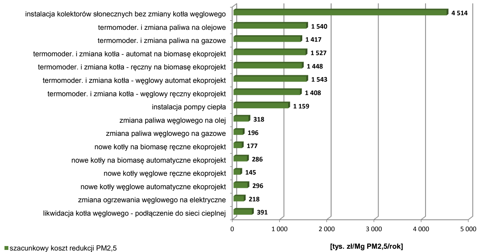
Rysunek 17. Porównanie szacunkowych, średnich wskaźników kosztów redukcji pyłu zawieszzonego PM2,5 z indywidualnych systemów grzewczych
