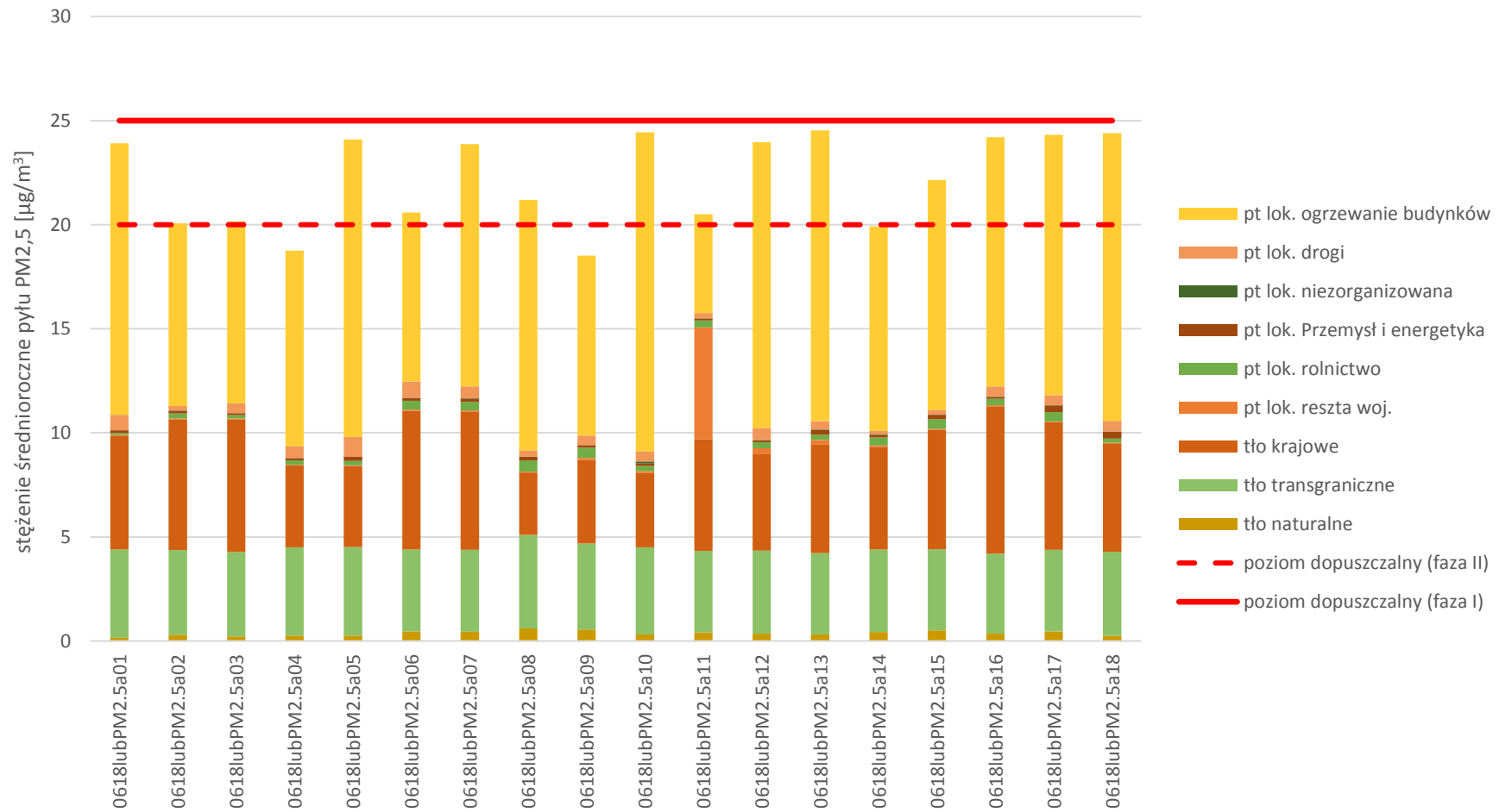
Rysunek 14. Prezentacja poziomów tła regionalnego oraz przyrostu tła lokalnego na terenie obszarów przekroczeń pyłu PM2,5 w strefie lubelskiej w 2018 roku
