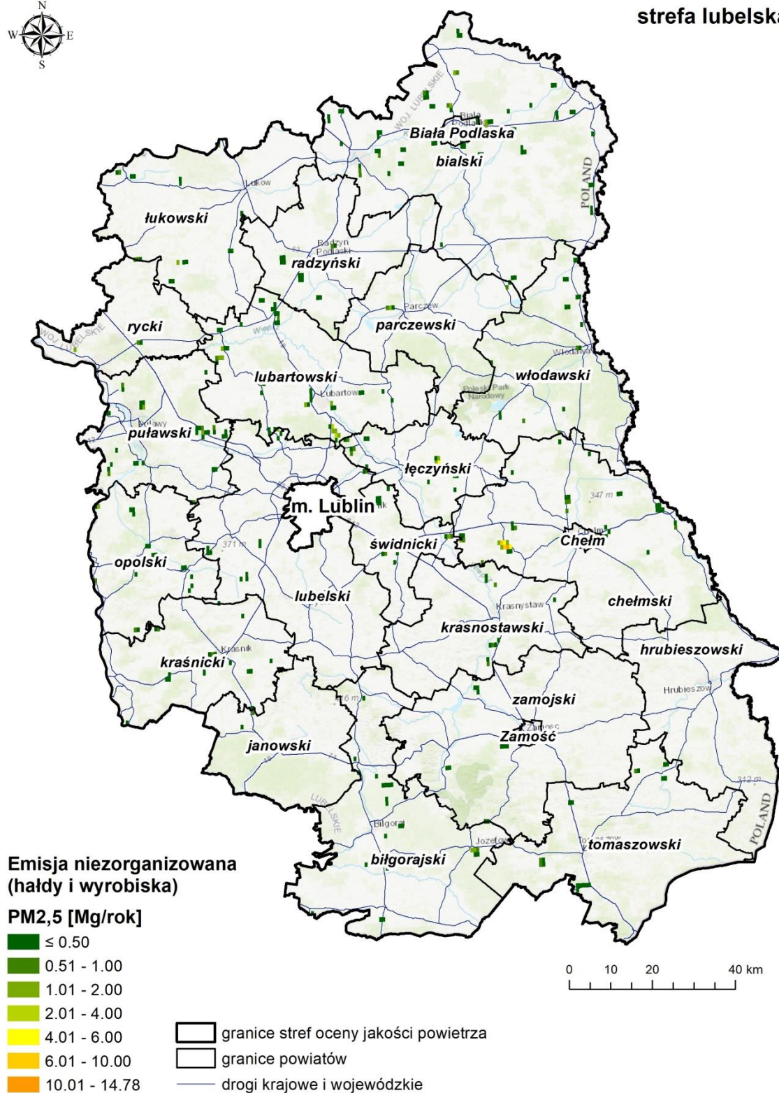
Rysunek 36. Emisja pyłu zawieszonego PM2,5 ze źródeł niezorganizowanych (hałdy i wyrobiska) 91
