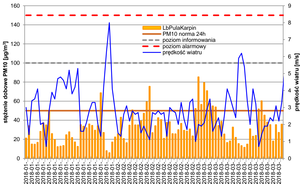
Rysunek 6. Przebieg zmienności stężeń 24-godz. PM10 w 2018 r. oraz prędkości wiatru w pierwszym kwartale 2018 roku w strefie lubelskiej w Puławach 43
