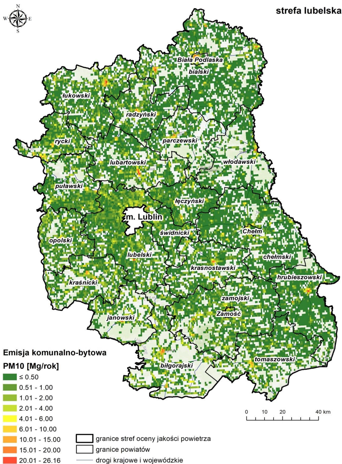
Rysunek 47. Emisja pyłu zawieszonego PM10 z sektora komunalno-bytowego 102
