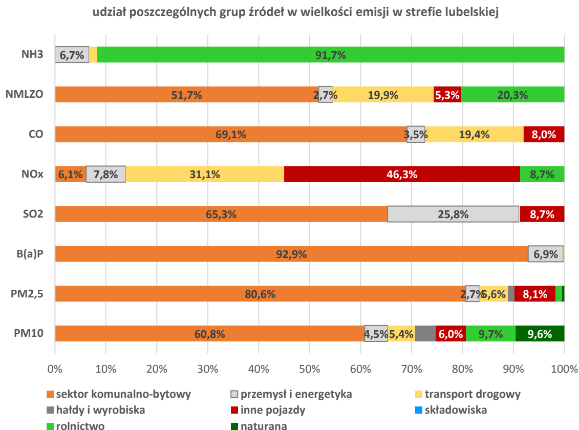
Rysunek 12. Udział poszczególnych grup źródeł emisji w bilansie zanieczyszczeń wprowadzanych do powietrza w strefie lubelskiej w 2018 roku
