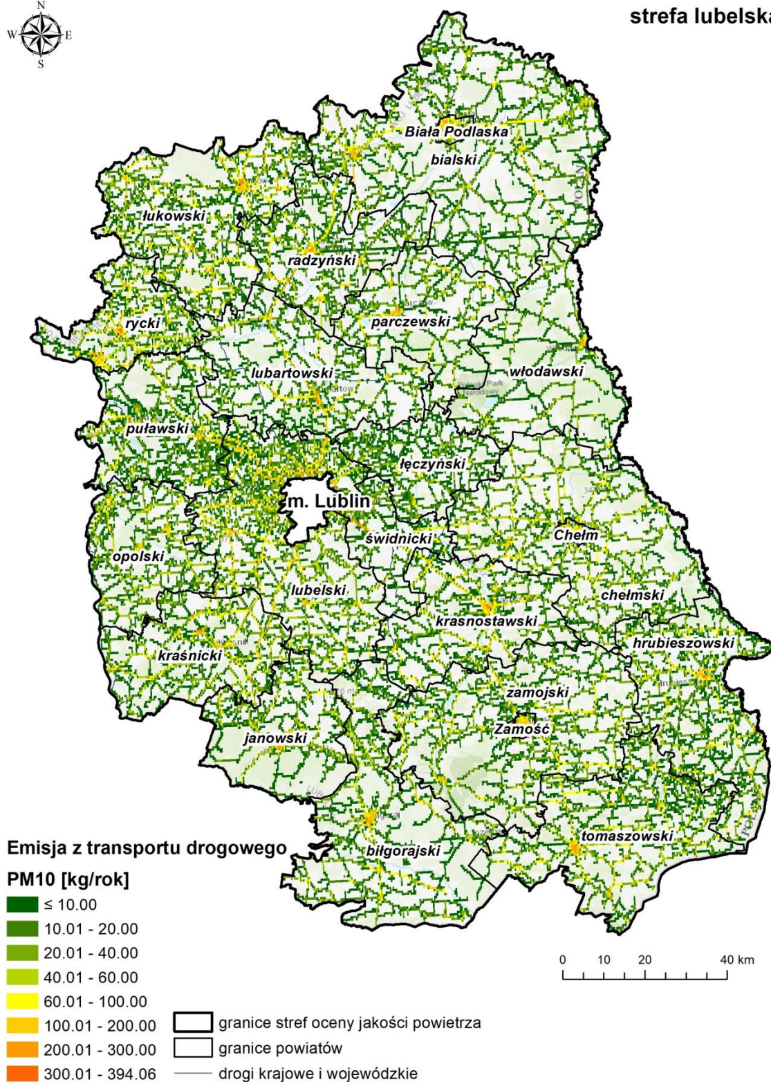
Rysunek 28. Emisja pyłu zawieszonego PM10 z transportu drogowego 83
