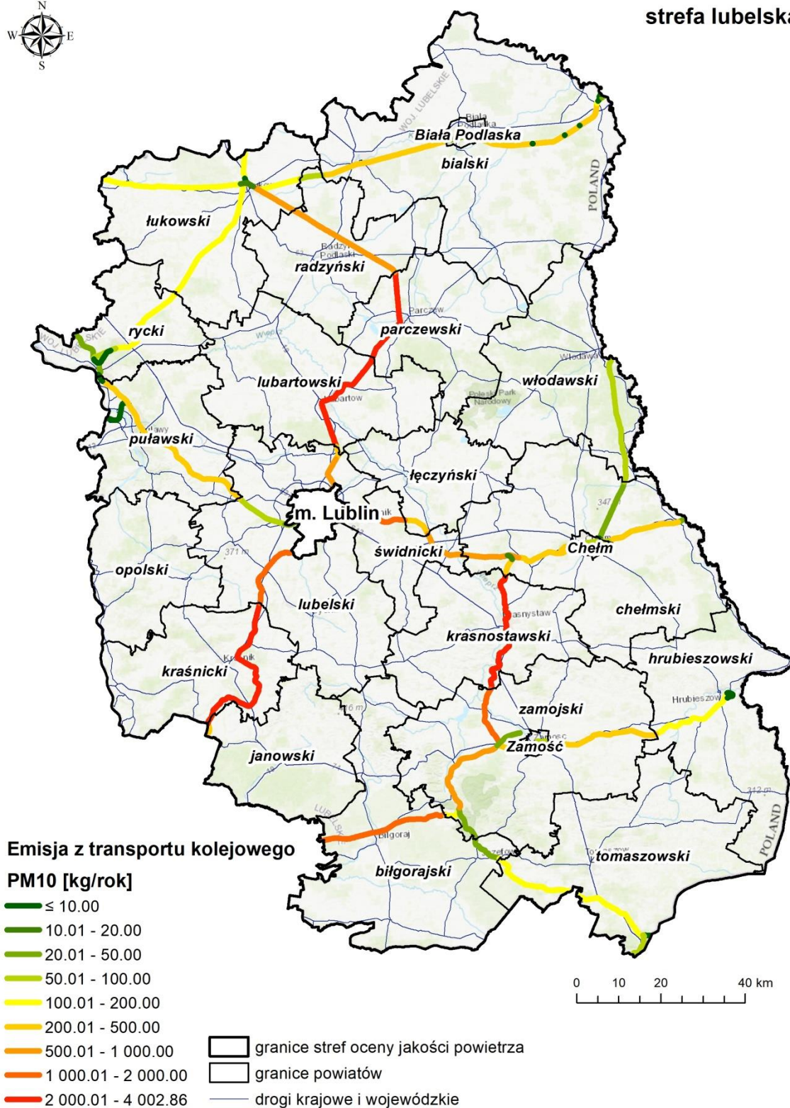
Rysunek 30. Emisja pyłu zawieszonego PM10 z innych źródeł (kolej) 85
