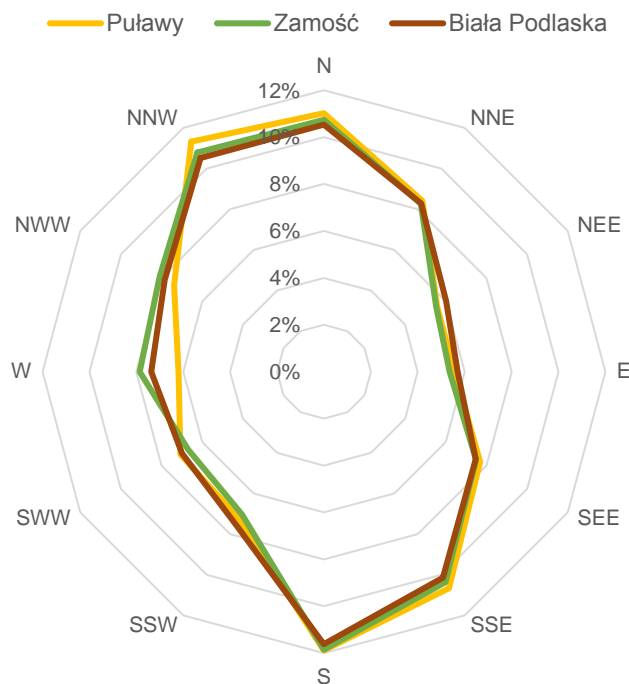
Rysunek 2. Róża wiatrów w strefie lubelskiej w 2018 roku, na podstawie danych stacji pomiarowej w Puławach, Zamościu i Białej Podlaskiej 29
