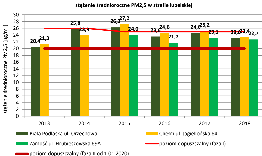
Rysunek 7. Stężenie średnioroczne PM 2,5 w strefie lubelskiej za lata 2013-2018 44
