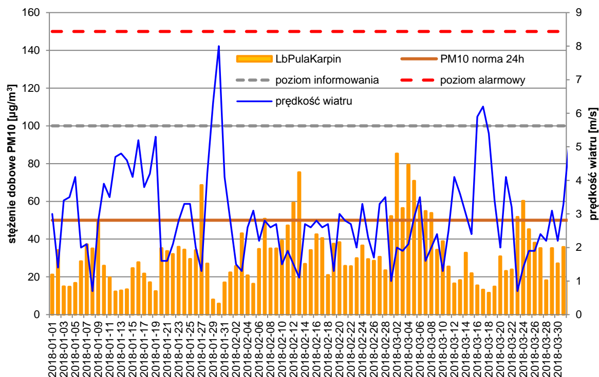
Rysunek 18. Porównanie przebiegu zmienności stężeń 24-godz. PM10 w I kwartale 2018 r. w Puławach z prędkością wiatru
