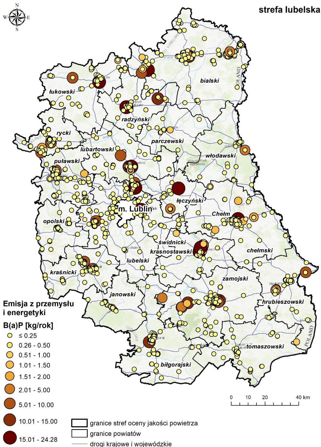
Rysunek 44. Emisja benzo(a)pirenu ze źródeł przemysłowych i energetycznych 99
