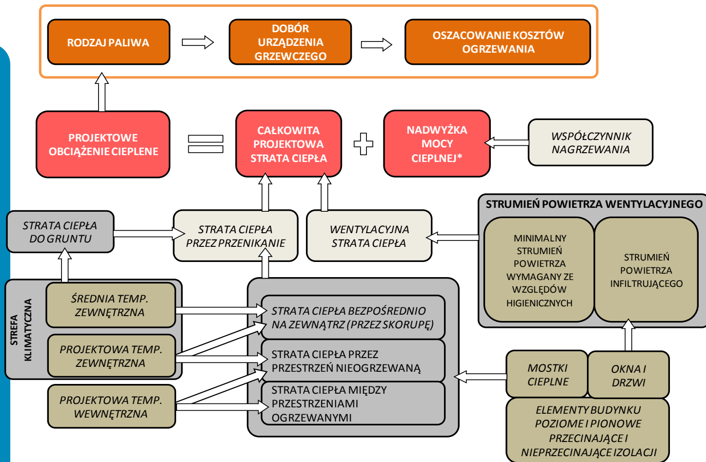
Rys. 18. Wielkości wpływające na dobór rodzaju i wielkości urządzenia grzewczego
