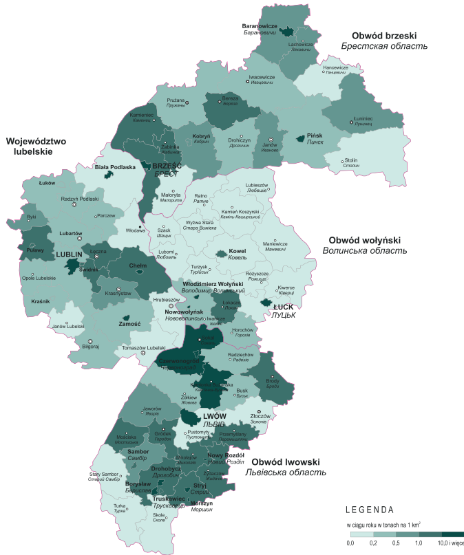
Ryc. 2.9. Emisja przemysłowych, pyłowych i gazowych zanieczyszczeń powietrza atmosferycznego w 2011 r.
