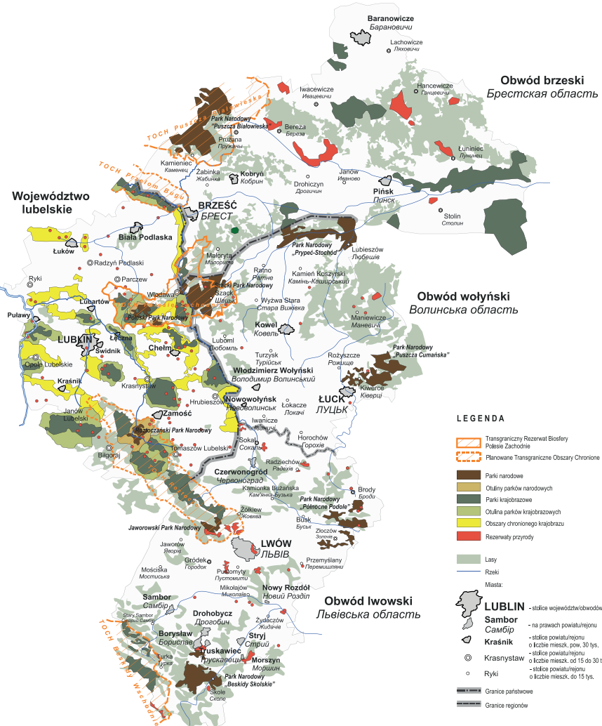
Ryc. 2.7. Formy ochrony przyrody
