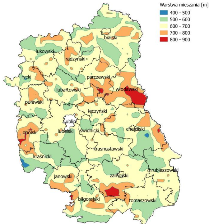
Rysunek 14 Rozkład średniej rocznej wysokości warstwy mieszaniny wyznaczony przez model WRF/CALMET w strefie lubelskiej w 2015 r.
